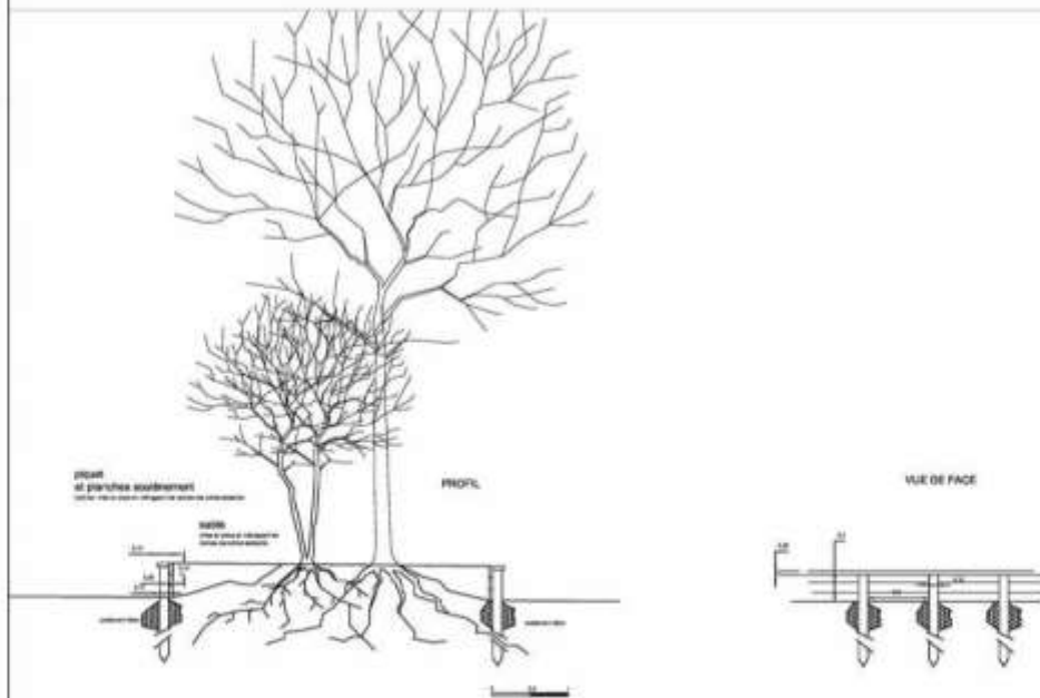
DETAIL 12 bac à sable arboré (profil)
